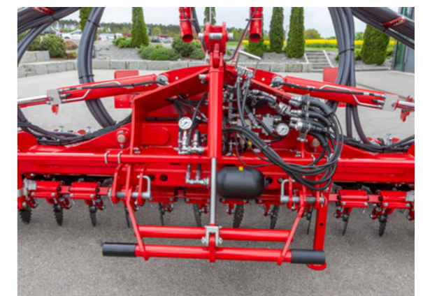
Avatar SL – hydraulický přenos hmotnosti pro přenos dodatečné síly
