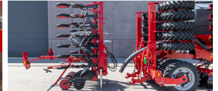
Rampes de semis facilement interchangeables grâce à l'attelage 3 points
