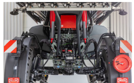
Hintereinander liegende Schiebeachsen und hydropneumatische Federung
