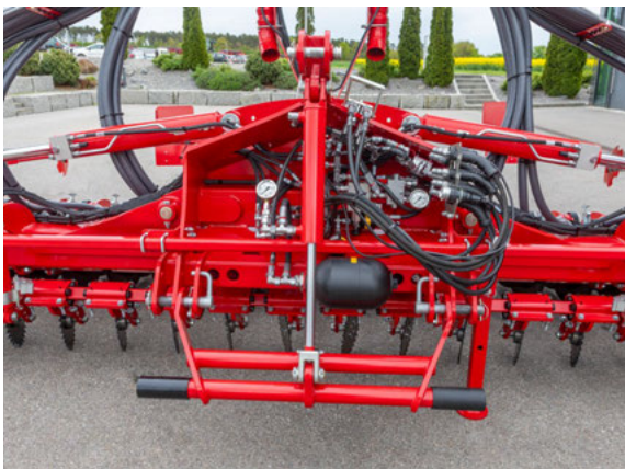
Avatar SL – report de charge hydraulique pour application d'une pression maximale
