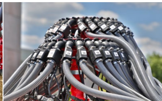
En las versiones de doble torre se puede elegir entre el cierre de media anchura o la manguera selectiva
