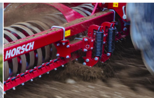
Spurlockerzinken lösen Spuren auf
