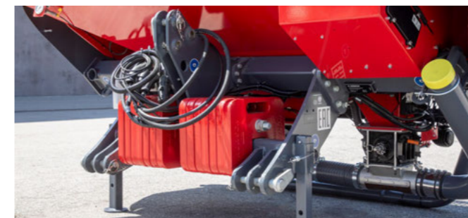
Perfektní rovnováha díky přidávným závažím
