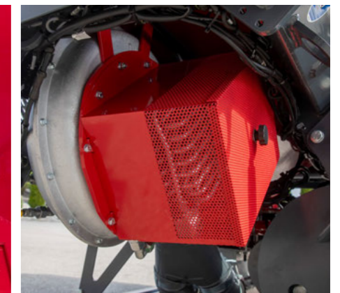
Volitelný olejový chladič pro ohřev nasávaného vzduchu
